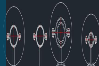
丙二醇 Ø51X1.5 保温50mm 麦汁 Ø51X1.5 蒸汽 Ø54X4 保温50mm 冷凝水 Ø31X3 保温50mm
